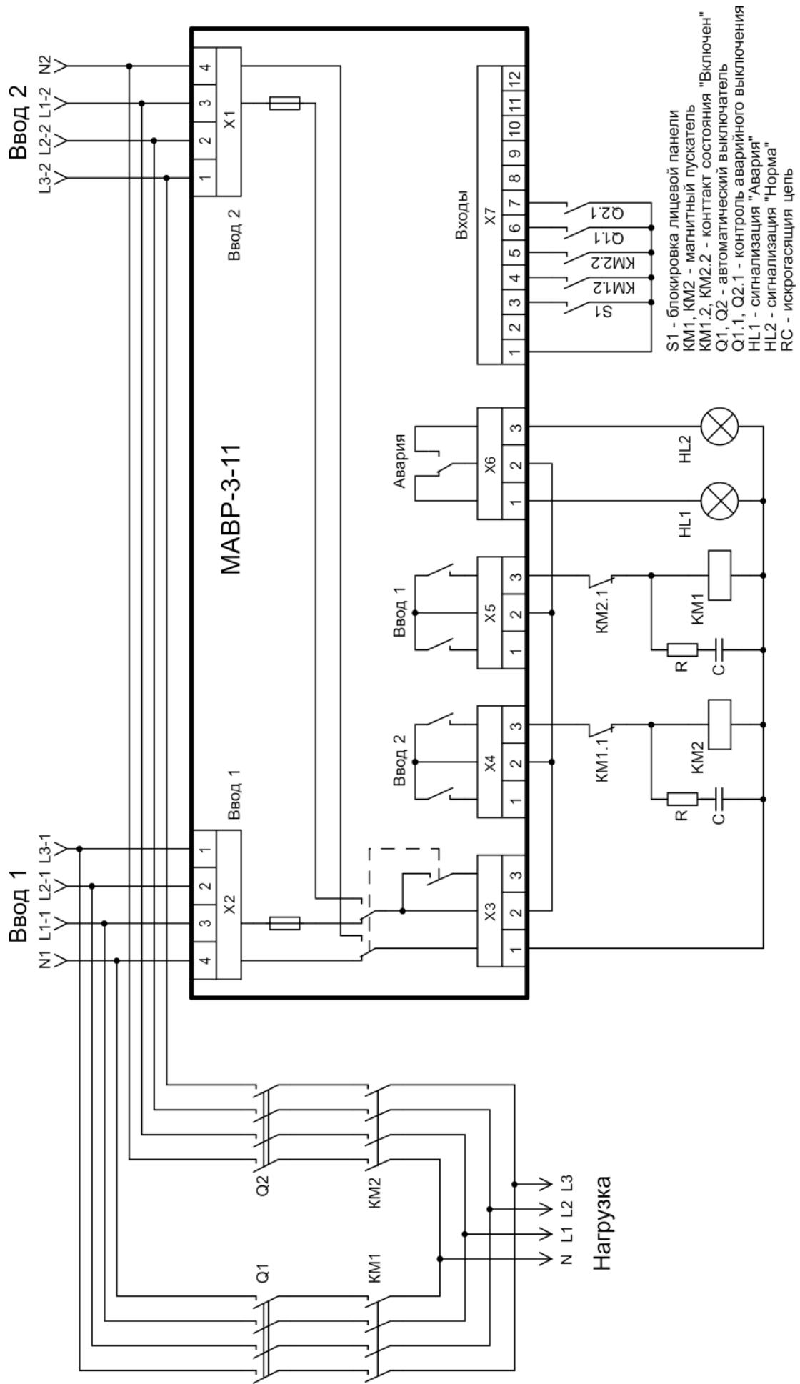
Рис. 7. Подключение нагрузки магнитными пускателями
