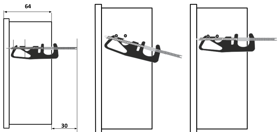
Рис. 5. Порядок установки
